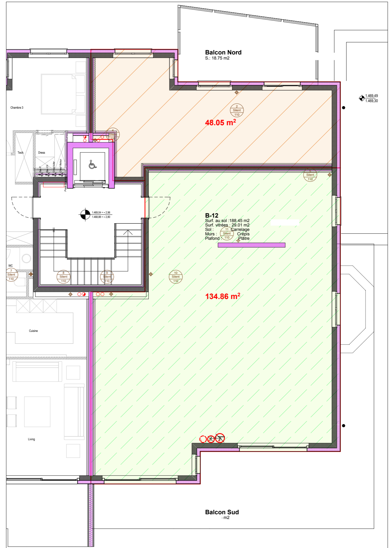
1. Niveau 1 1:100
